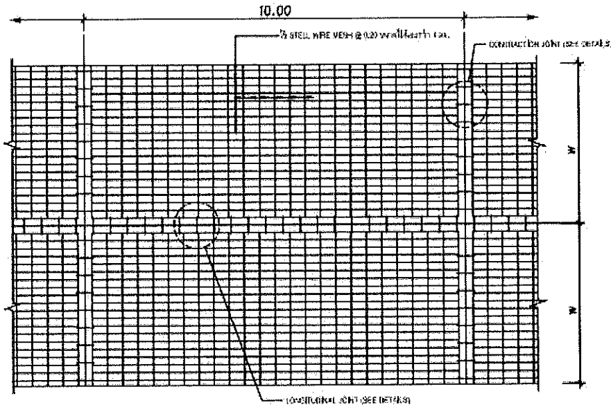
PLAN แสดงการเสริมเหล็กใน CONCRETE PAVEMENT
